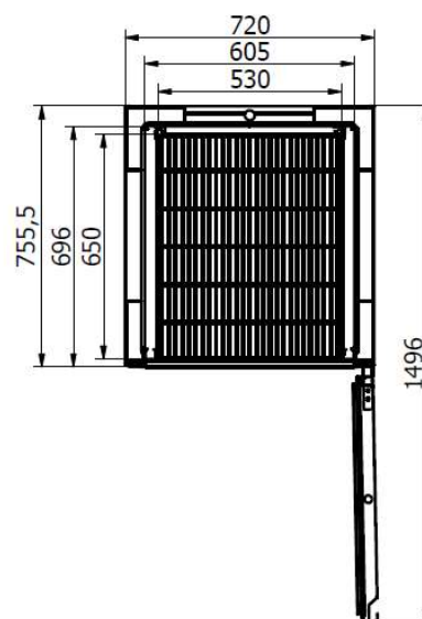
Vue de haut porte ouverte
